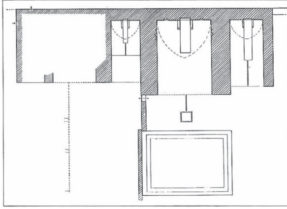
Firdevs Köşkü planı
