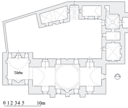
Melik Mansur Medresesi Planı (M. Baran Arşivi'nden)
