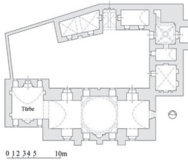
Melik Mahmud Cami Planı (M. Baran Arşivi'nden)
